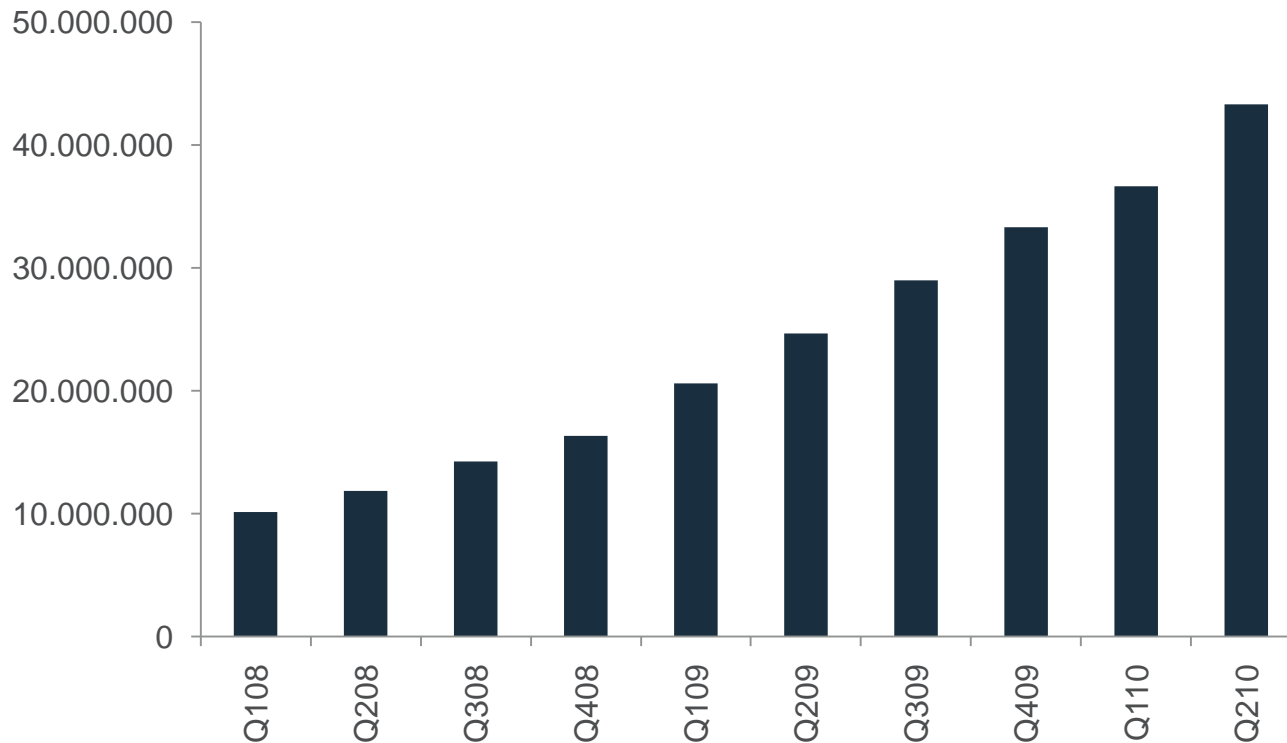
Anzahl der Malware Samples in der McAfee Datenbank
